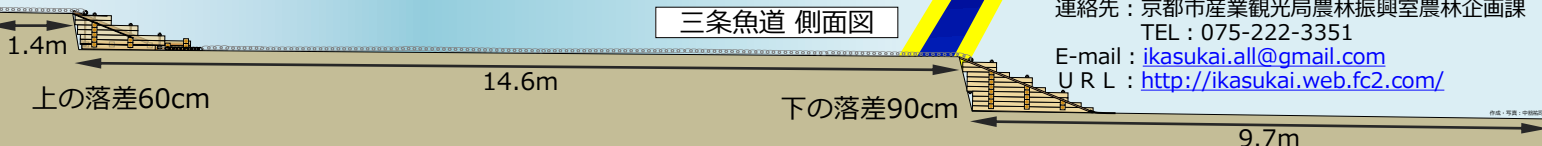
平成30年4月28日 三条落差工で魚道の設置活動
