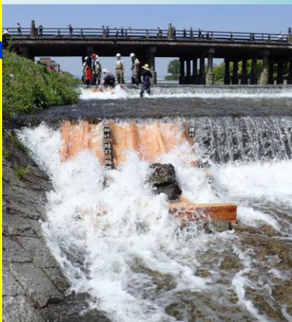
平成30年4月28日 三条落差工で魚道の設置活動
